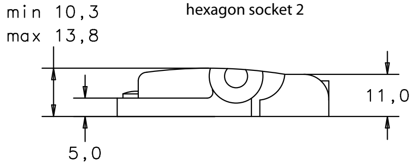
Vorderansicht front view
