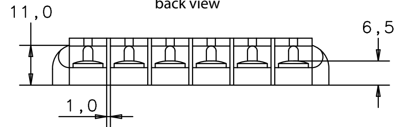
Rückansicht back view
