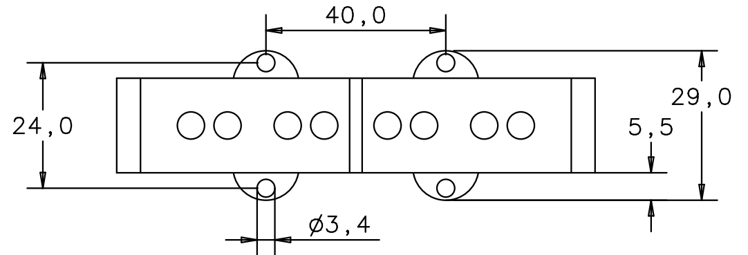
Unteransicht bottom view
