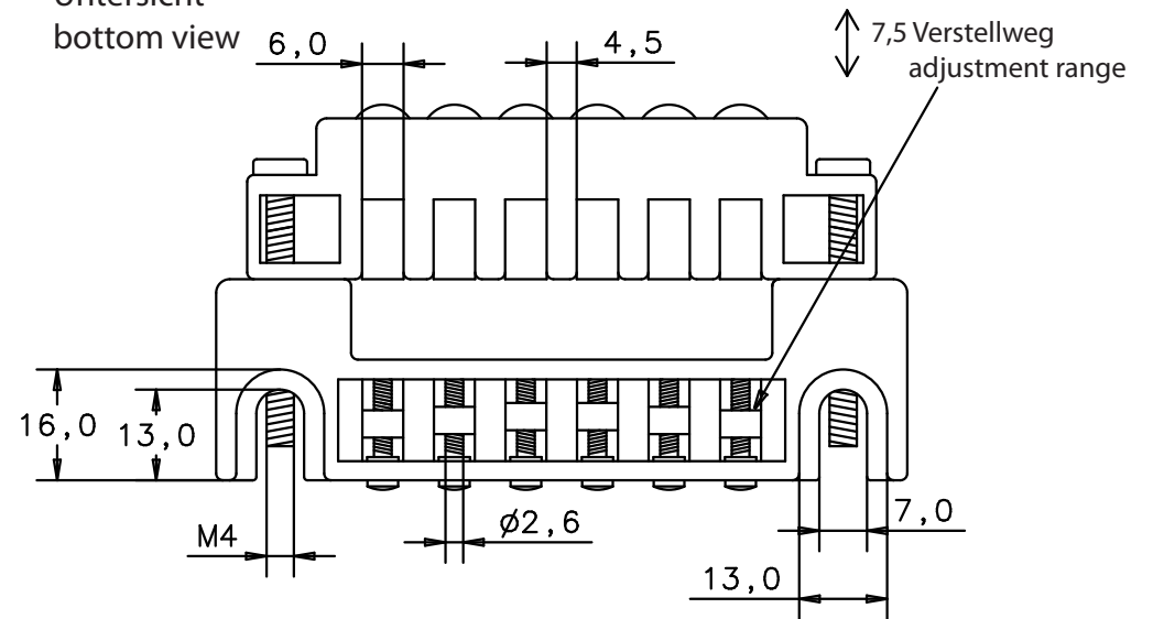
Einschlagmutter insert
