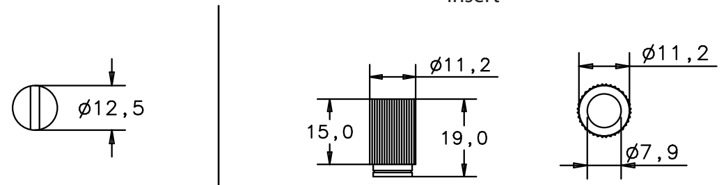
Einschlagmutter insert
