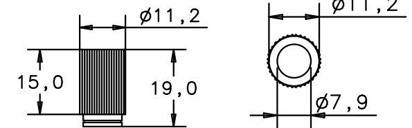
Einschlagmutter insert
