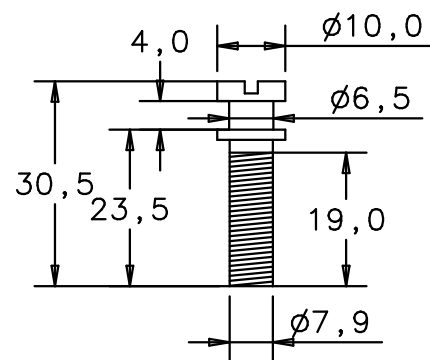
Höhenverstellerschraube level adjustable screw
