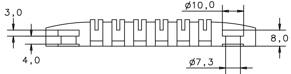
Untersicht bottom view
