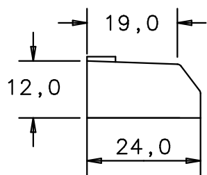
Seitenansicht side view
