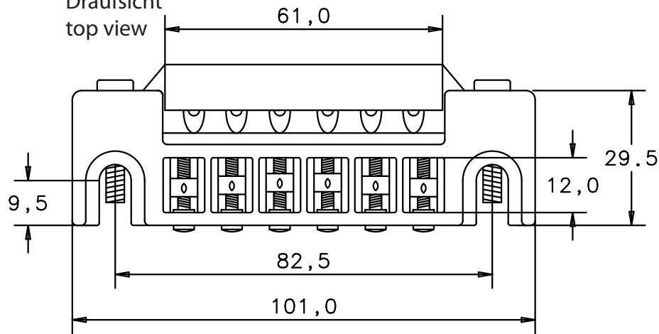
Höhenverstellerschraube level adjustable screw
