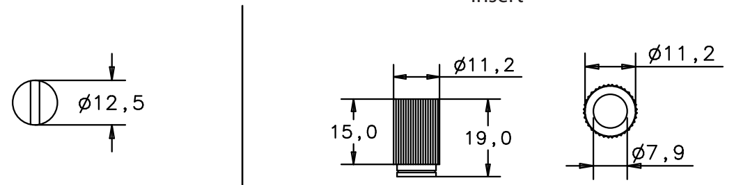
Einschlagmutter insert
