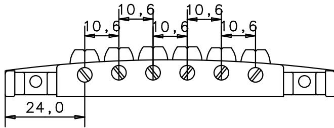
Vorderansicht front view
