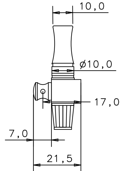
Seitenansicht von links side view left
