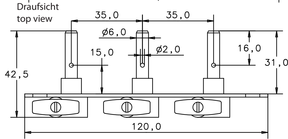
Gegenlager thrust bearing
