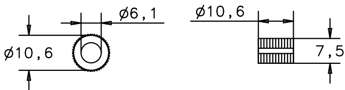
Gegenlager thrust bearing
