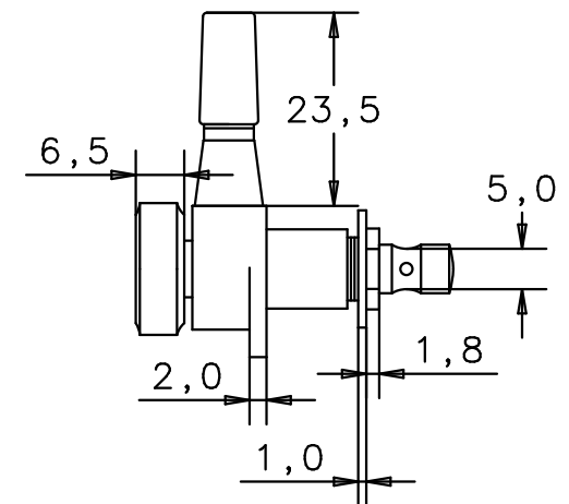
Seitenansicht von rechts side view right
